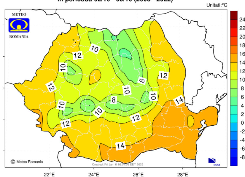
Media multianuala a temperaturii aerului la 2 m in perioada 02/10 - 09/10 (2003 - 2022)
