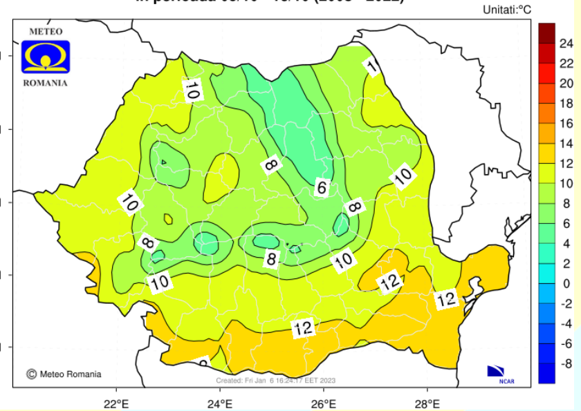
Media multianuala a temperaturii aerului la 2 m in perioada 09/10 - 16/10 (2003 - 2022)
